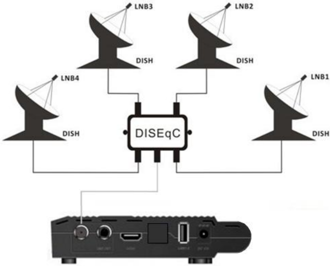
Şekil 7 Çanak LNB'sine bağlantı
